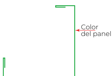
FLASHING ESQUINERO
